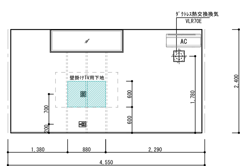
LDK 南面
