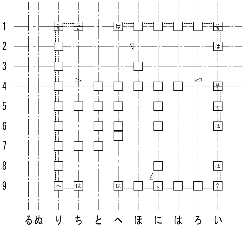
2階柱壁伏図
