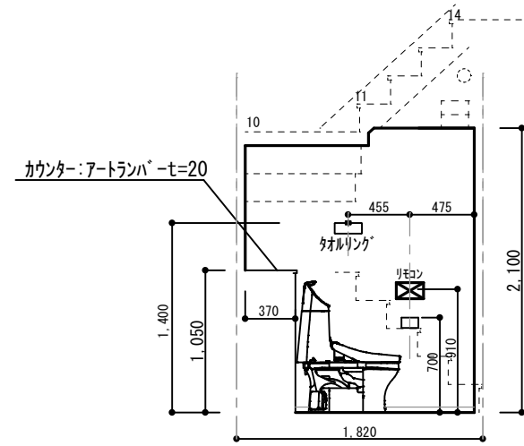
WC① 北面
