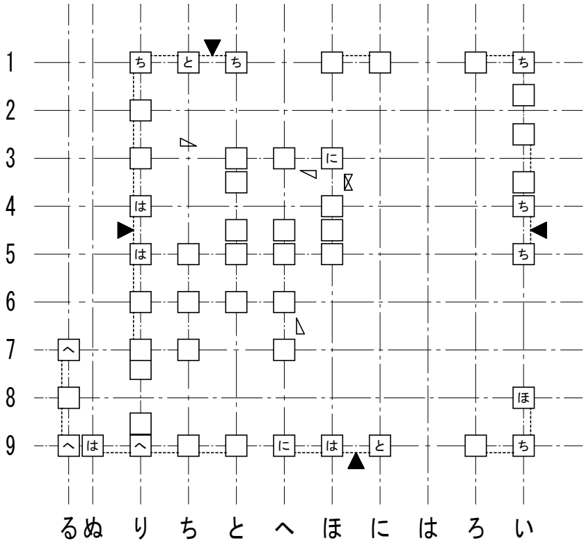
1階柱壁伏図
