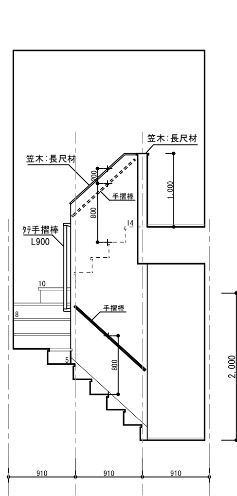
階段 北面
